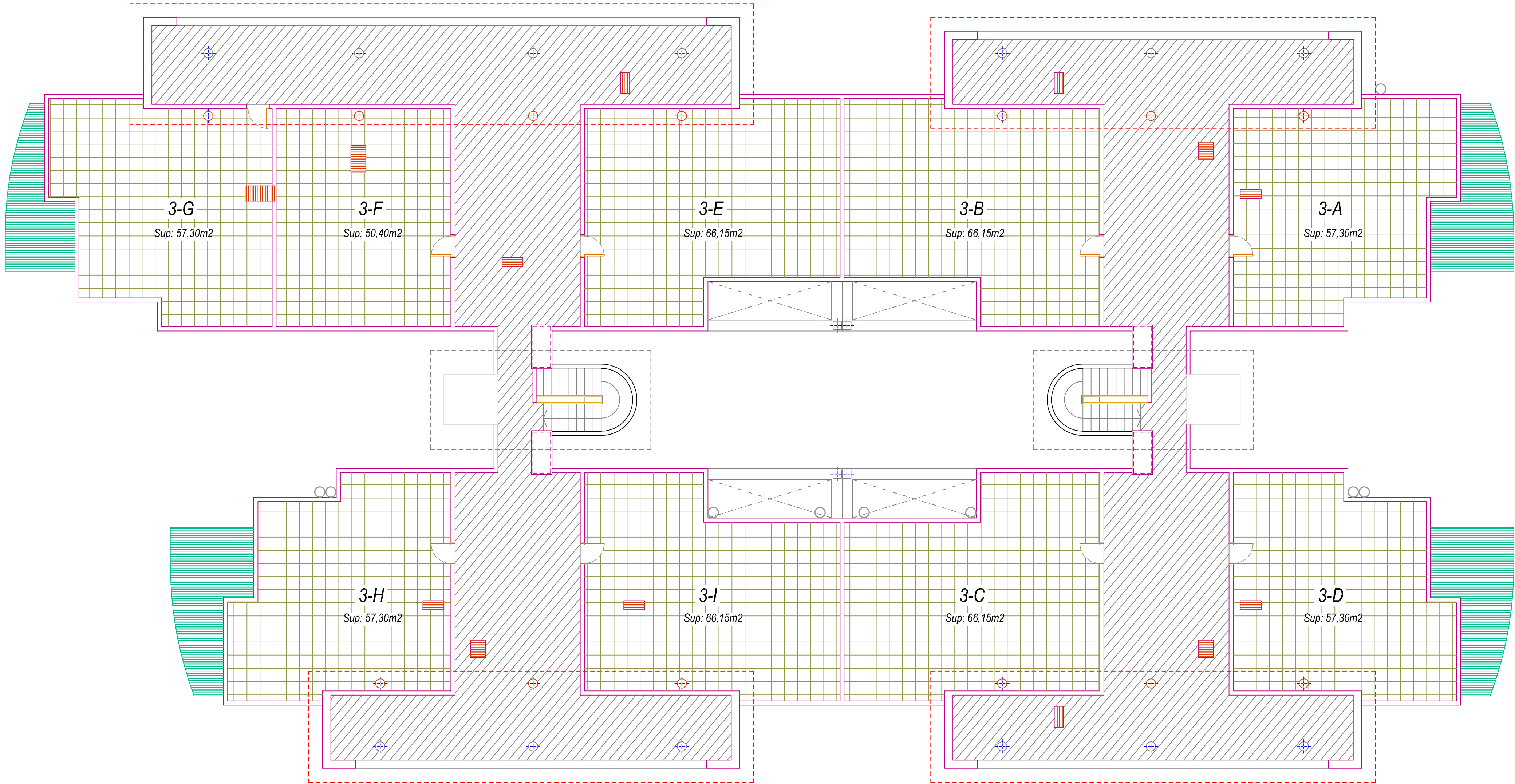
CUBIERTA BLOQUE 3
